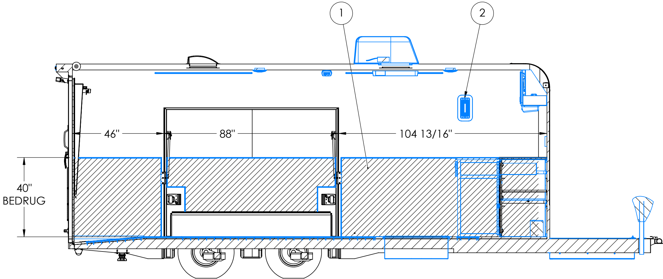
SECTION D-D SCALE 1 : 28
